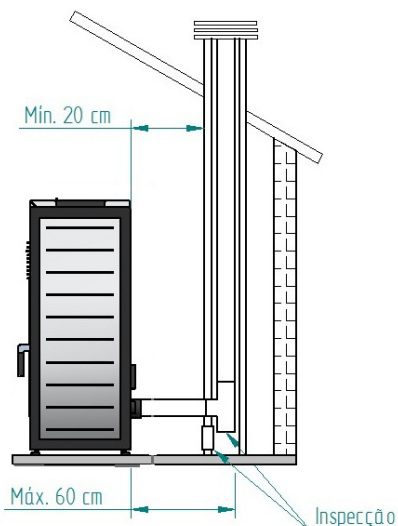
Figura 18 – Vista lateral da instalação com chaminé, com exemplo do ponto de inspeção
