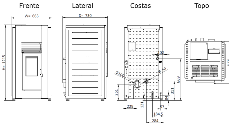
Figura 4 - Dimensões da salamandra a pellets (Douro 23 kW)
