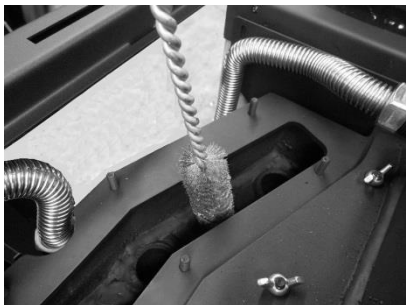
Figura 41 - Limpeza dos canais de passagem de ar e turbuladores
