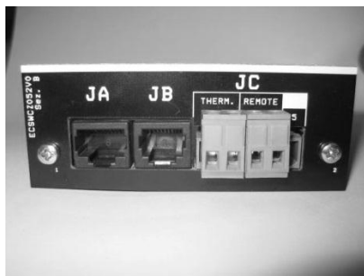
Figura 26 - Comando externo (cronotermostato) e interface de ligação – ambos não incluídos
