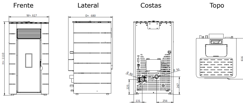
Figura 2 - Dimensões da salamandra a pellets (Douro 12 kW)
