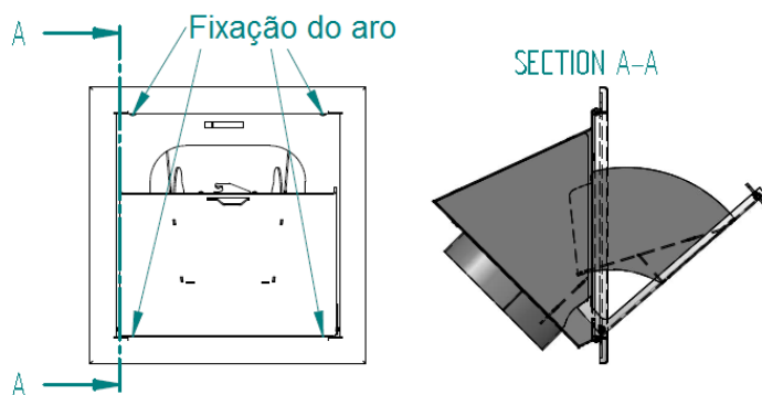
Figura 16 – Instalação equipamento
