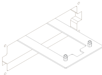
Figura 23 – Instalação do display fora do equipamento
