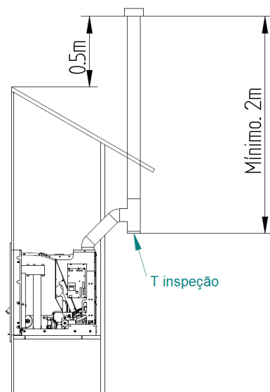
Figura 40 – Vista lateral da instalação sem chaminé, com exemplo do ponto de inspeção
