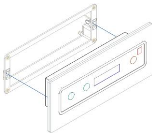
Figura 25 – Instalação do display fora do equipamento
