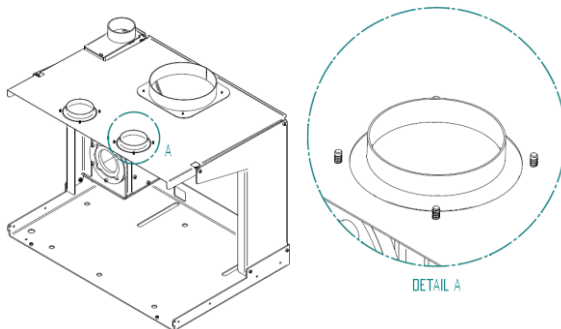
Figura 18 – Instalação inserível a pellets
