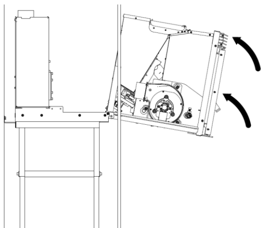
Figura 8 – Instalação
