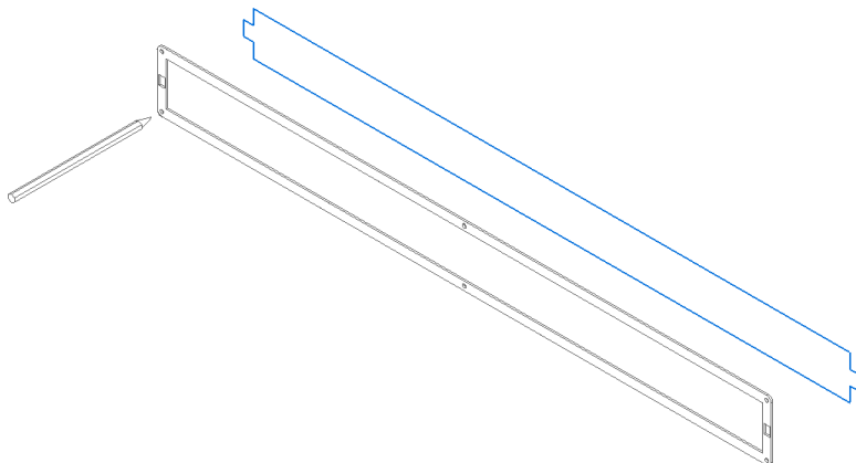
Figura 28 – Colocação acessórios
