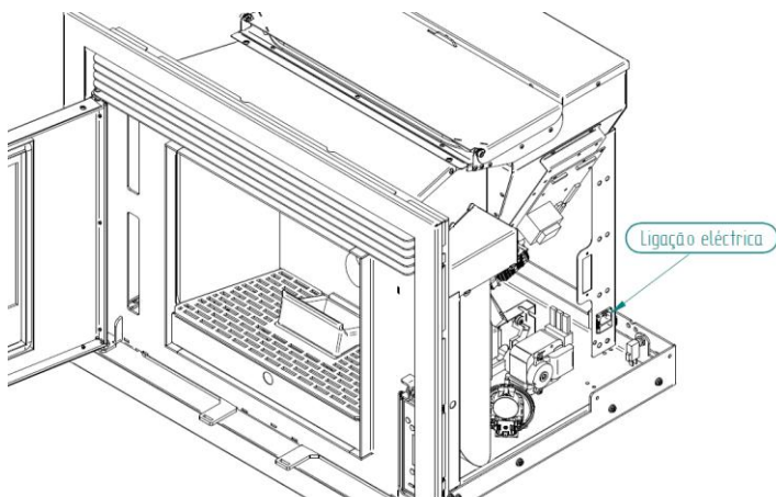
Figura 10 – Ligação elétrica
