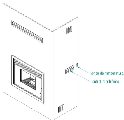
Figura 26 – Colocação acessórios
