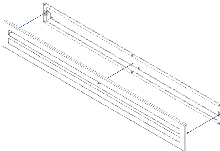
Figura 31 – Colocação acessórios
