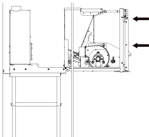
Figura 9 – Instalação
